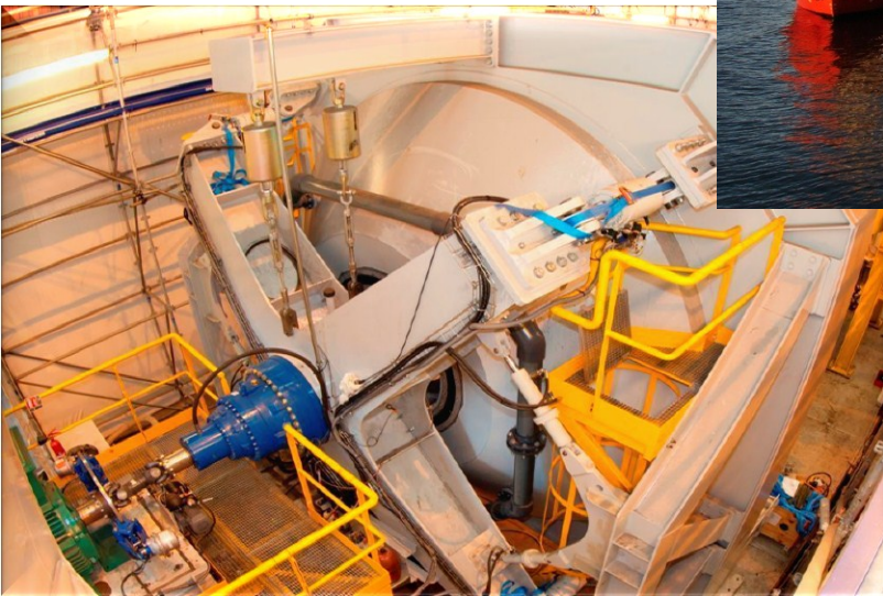
Alstom tidal test rig – Nantes, France
